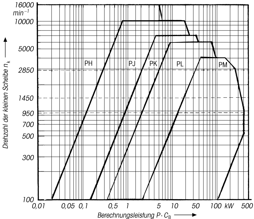
Diagr. 27.3 Richtlinien für die Profilwahl von Keilrippenriemen DIN 7867 (nach Conti Tech)
