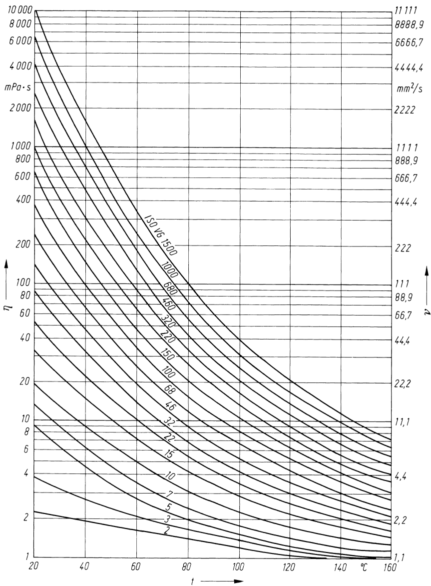
Diagr. 16.1 Dynamische Viskosität \eta in Abhängigkeit von der Temperatur t für Schmieröle (nach DIN 51519) mit der Dichte \rho = 900 \text{ kg/m}^3
